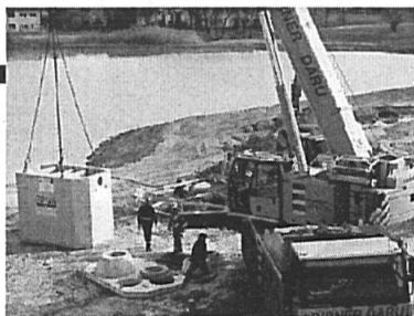
Környezetvédelmi víztisztító műtárgyak beépítése
